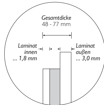
> Querschnitt der Türfüllung
